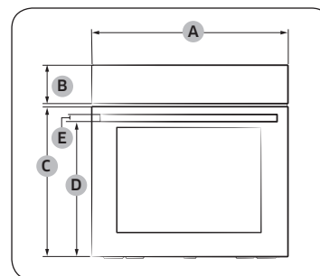
Piekarnik (mm)
