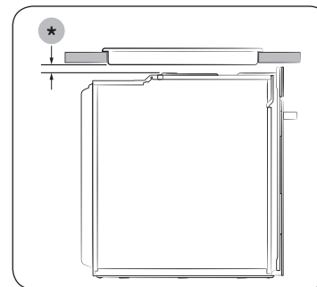
Montaż piekarnika
