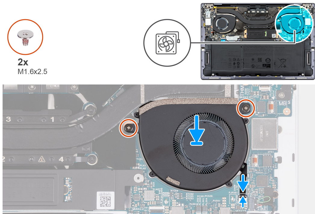
Rysunek 30. Instalowanie lewego wentylatora
