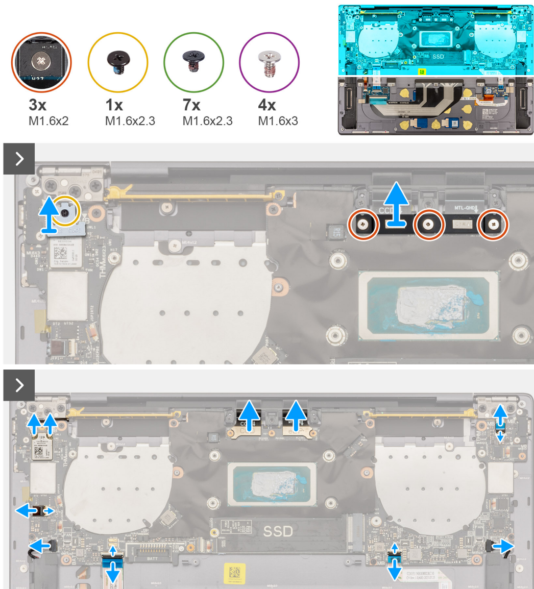
Rysunek 37. Wymontowywanie płyty głównej
