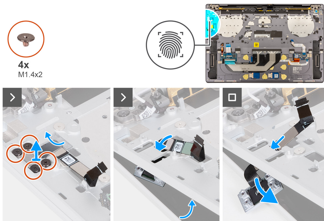
Rysunek 44. Wymontowywanie przycisku zasilania z czytnikiem linii papilarnych
