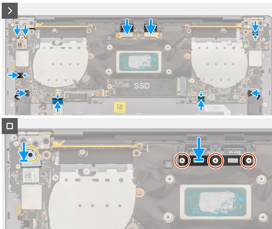
Rysunek 42. Instalowanie płyty głównej
