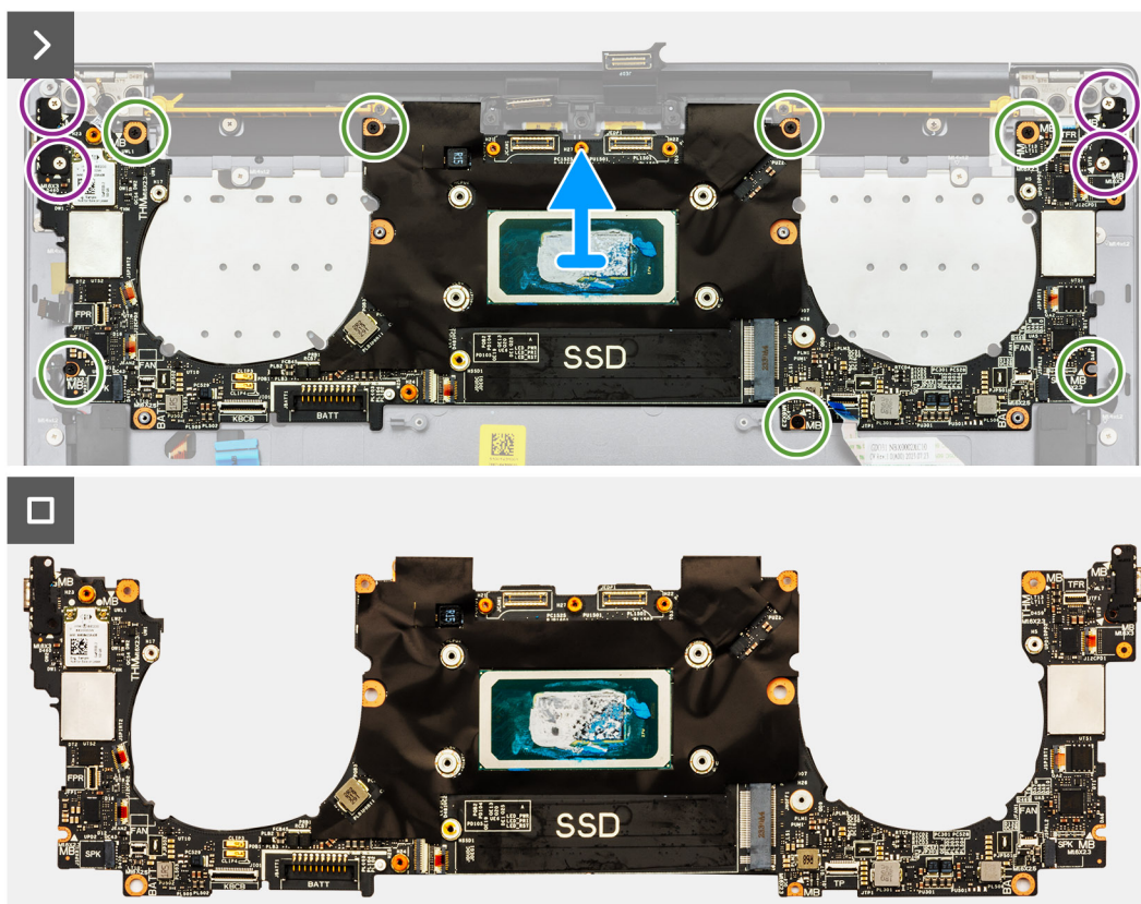
Rysunek 38. Wymontowywanie płyty głównej
