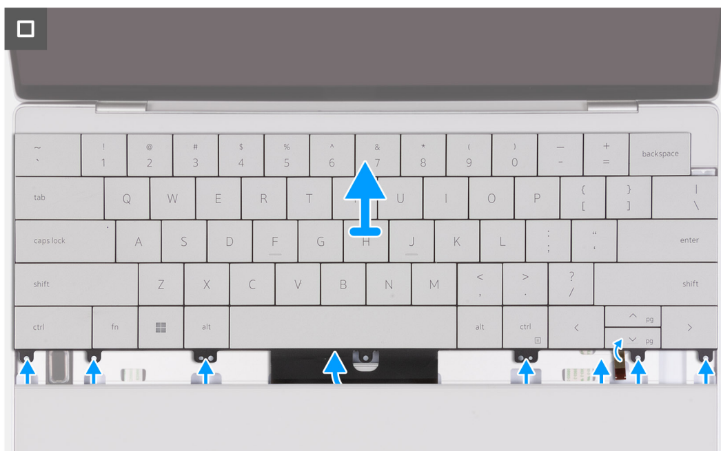
Rysunek 49. Wymontowywanie klawiatury
