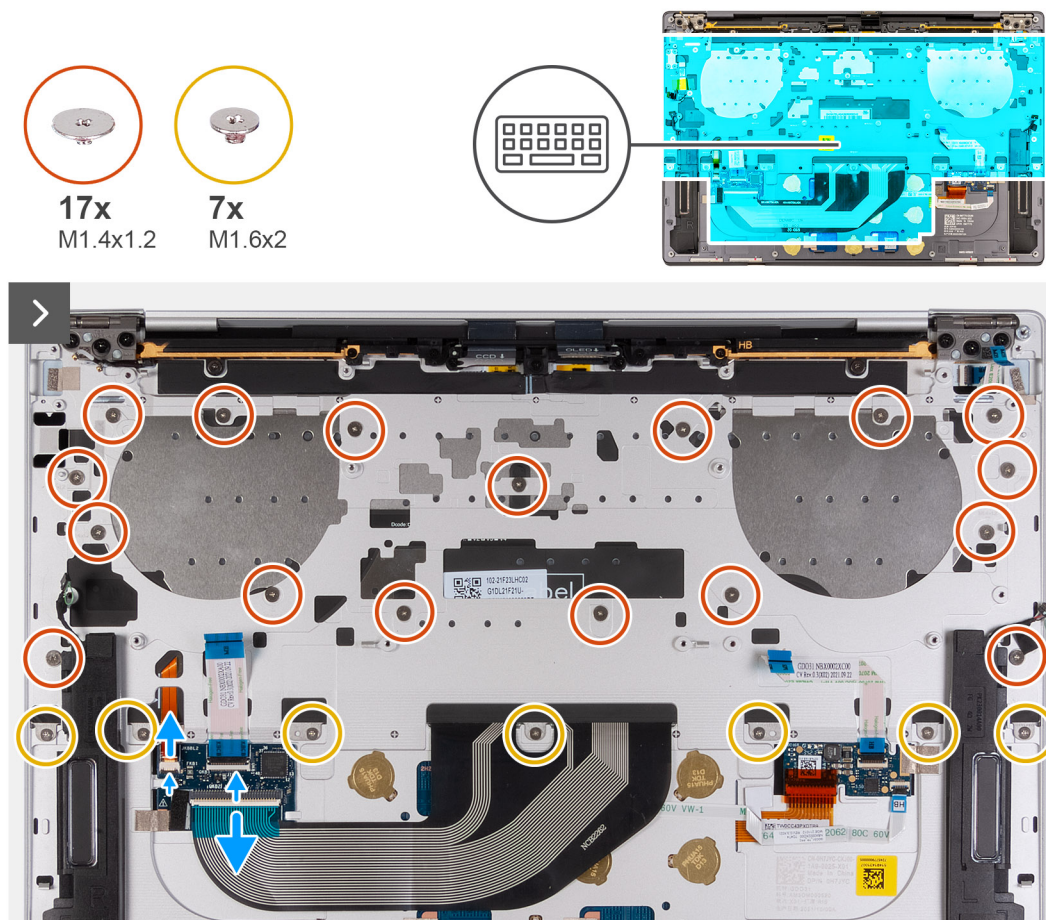
Rysunek 48. Wymontowywanie klawiatury
