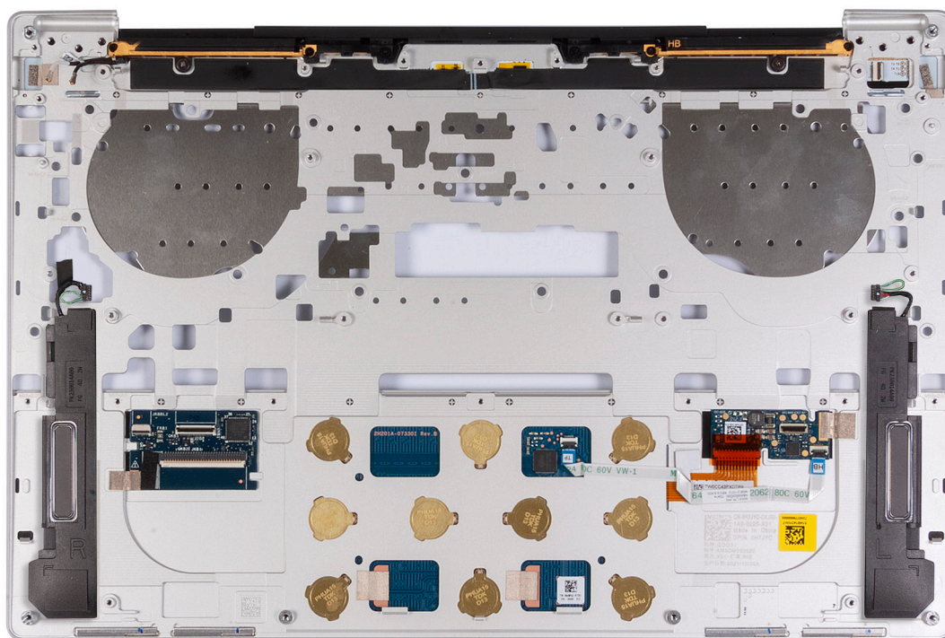
Rysunek 55. Instalowanie zestawu podpórki na nadgarstek
