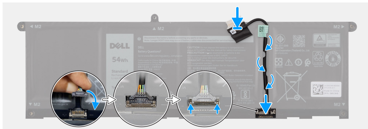
Rysunek 30. Podłączenie kabla baterii
