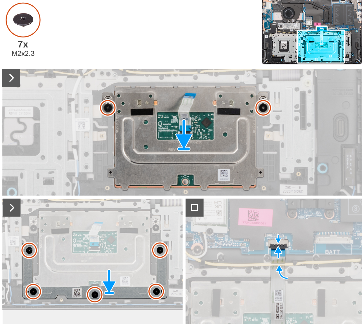
Rysunek 35. Instalowanie zestawu touchpada
