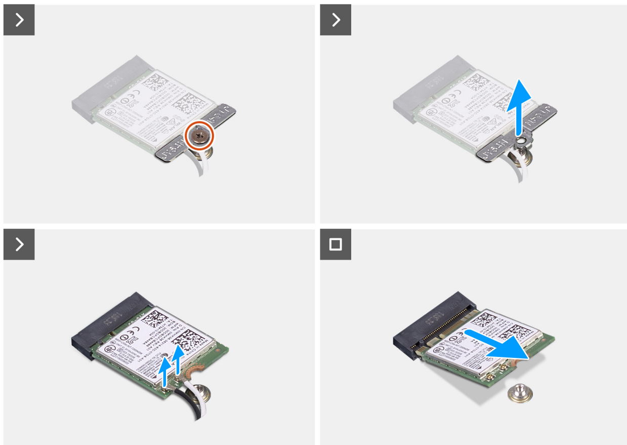
Rysunek 22. Wymontowywanie karty sieci bezprzewodowej
