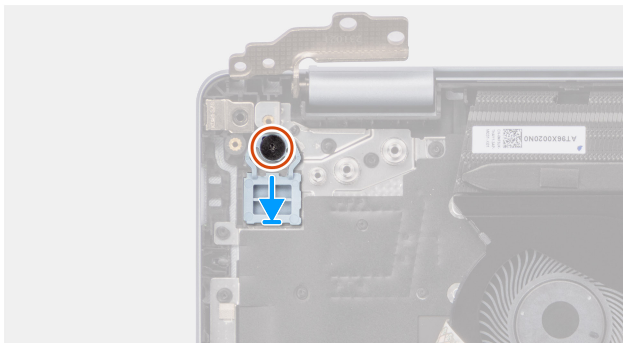
Rysunek 43. Instalowanie przycisku zasilania
