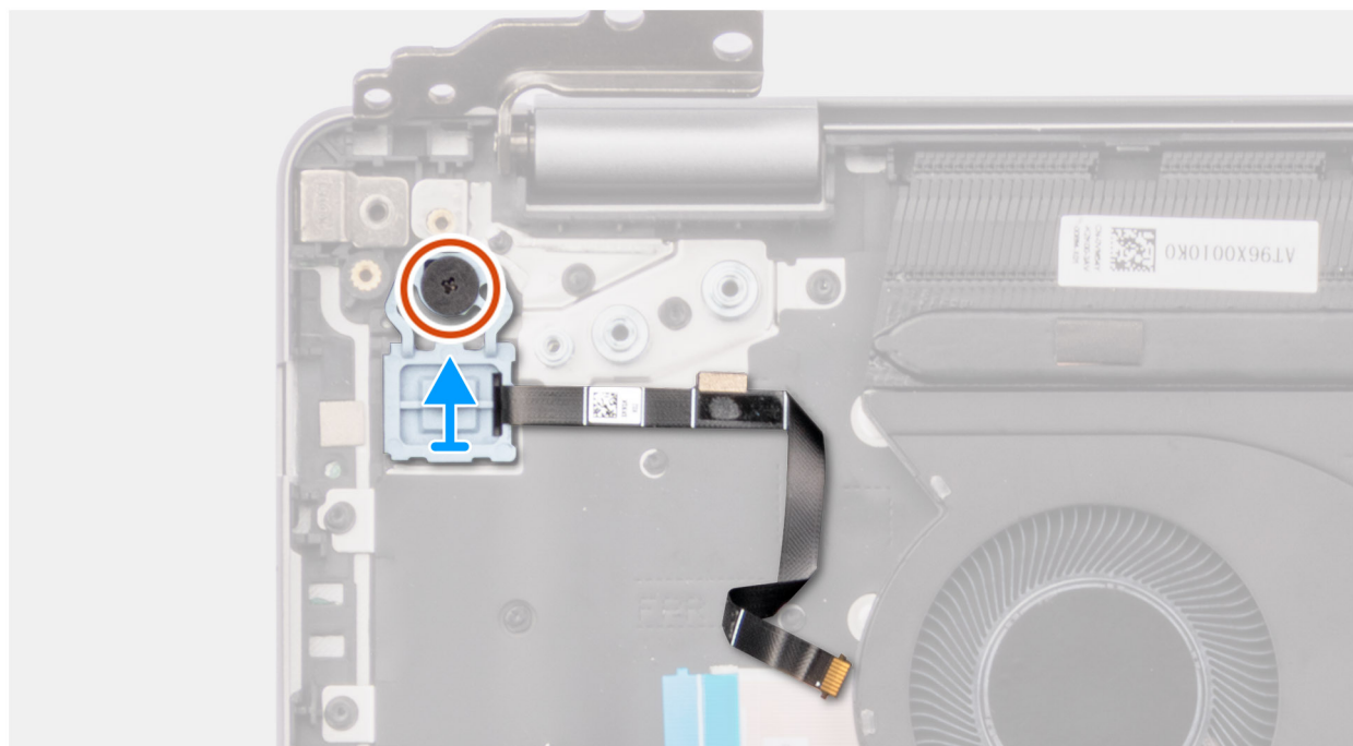
Rysunek 44. Wymontowywanie przycisku zasilania z opcjonalnym czytnikiem linii papilarnych
