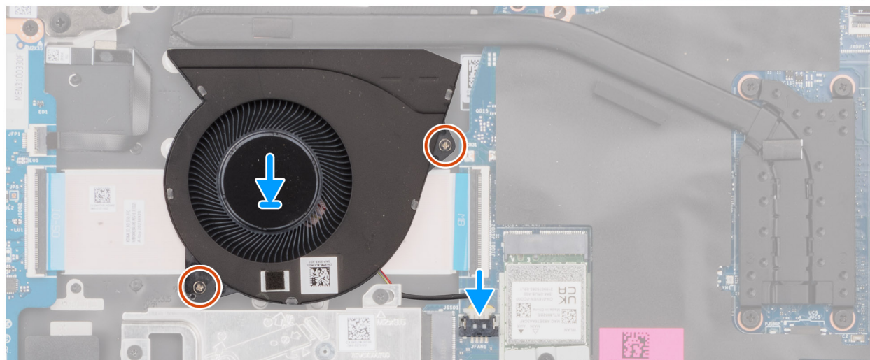
Rysunek 27. Instalowanie wentylatora
