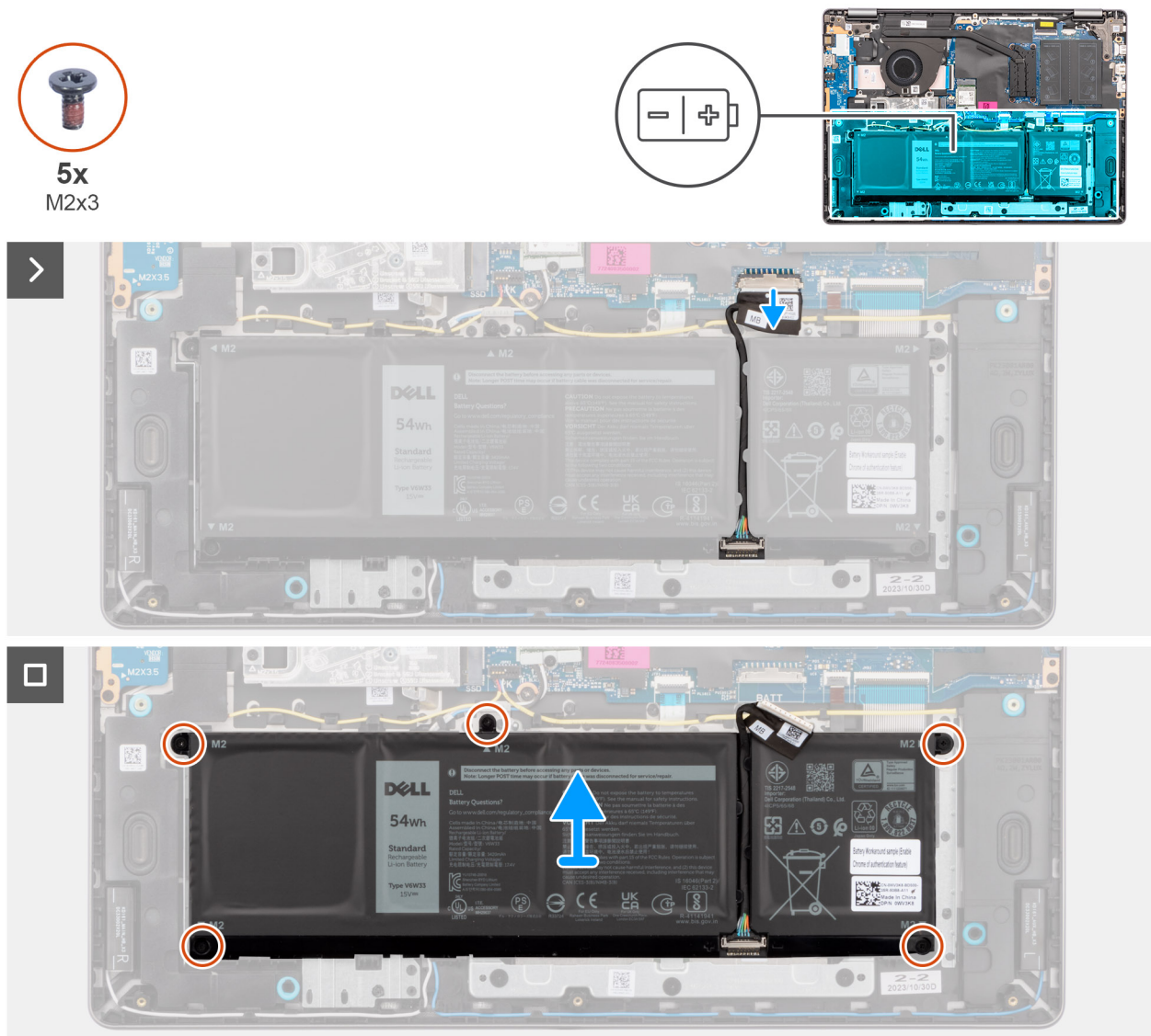
Rysunek 28. Wymontowywanie baterii
