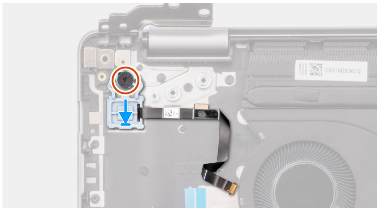
Rysunek 45. Instalowanie przycisku zasilania z opcjonalnym czytnikiem linii papilarnych
