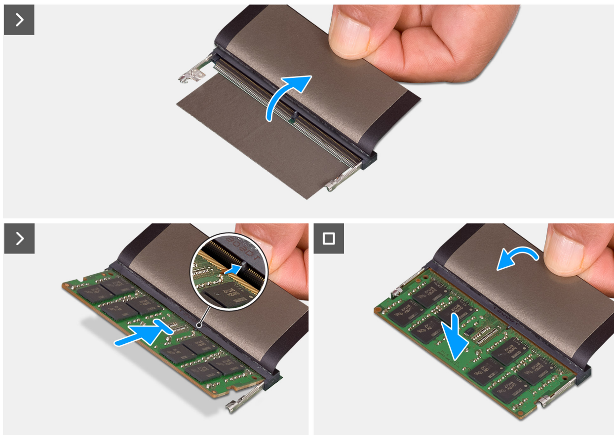
Rysunek 19. Instalowanie modułu pamięci
