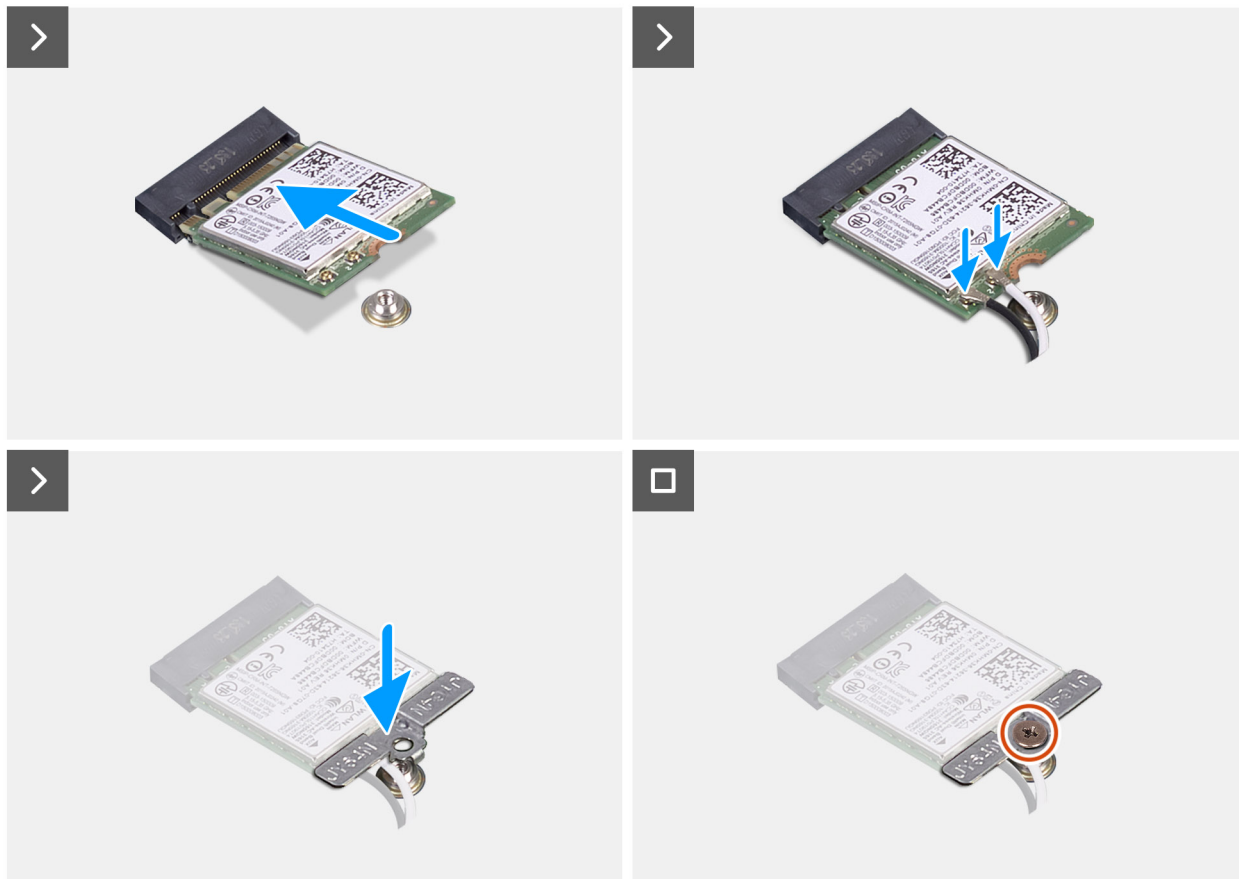
Rysunek 23. Instalowanie karty sieci bezprzewodowej
