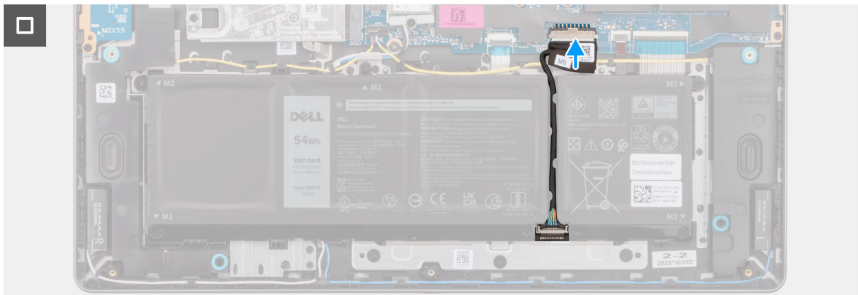
Rysunek 31. Instalowanie baterii
