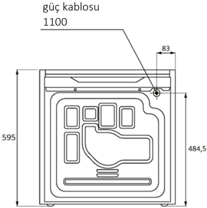
Arka görünüm
