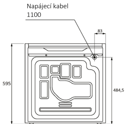
Pohled zezadu
