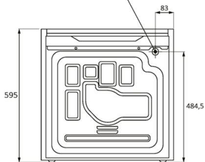
Οπίσθια όψη
