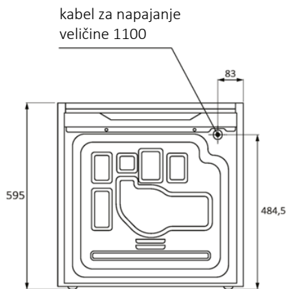
Pogled straga
