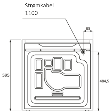
Set bagfra
