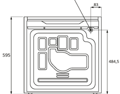
Vue arrière
