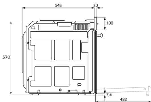
Изглед отстрани
