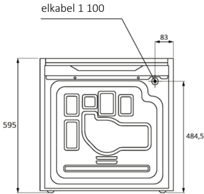
Baksida
