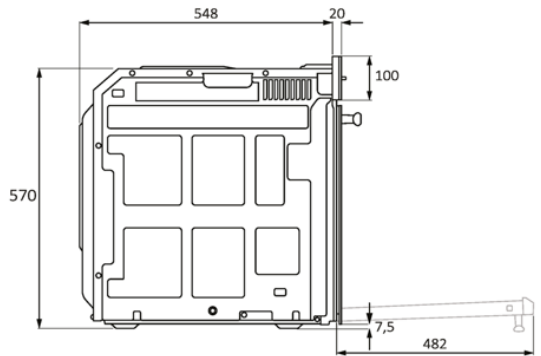
Seitenansicht
