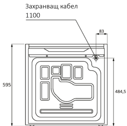
Изглед отзад
