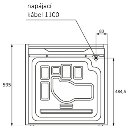
Pohľad zozadu
