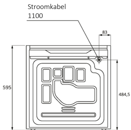
Achteraanzicht
