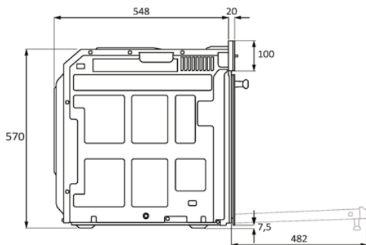
Vista laterale
